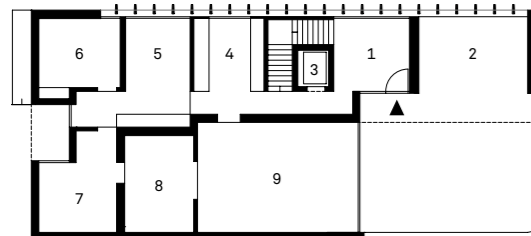
Untergeschoss M 1:400
